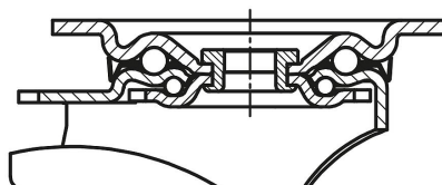
Forgócsapágyazás:
